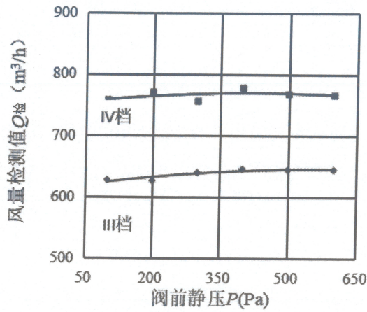
图 1 风量与阀前静压无关性检验曲线
